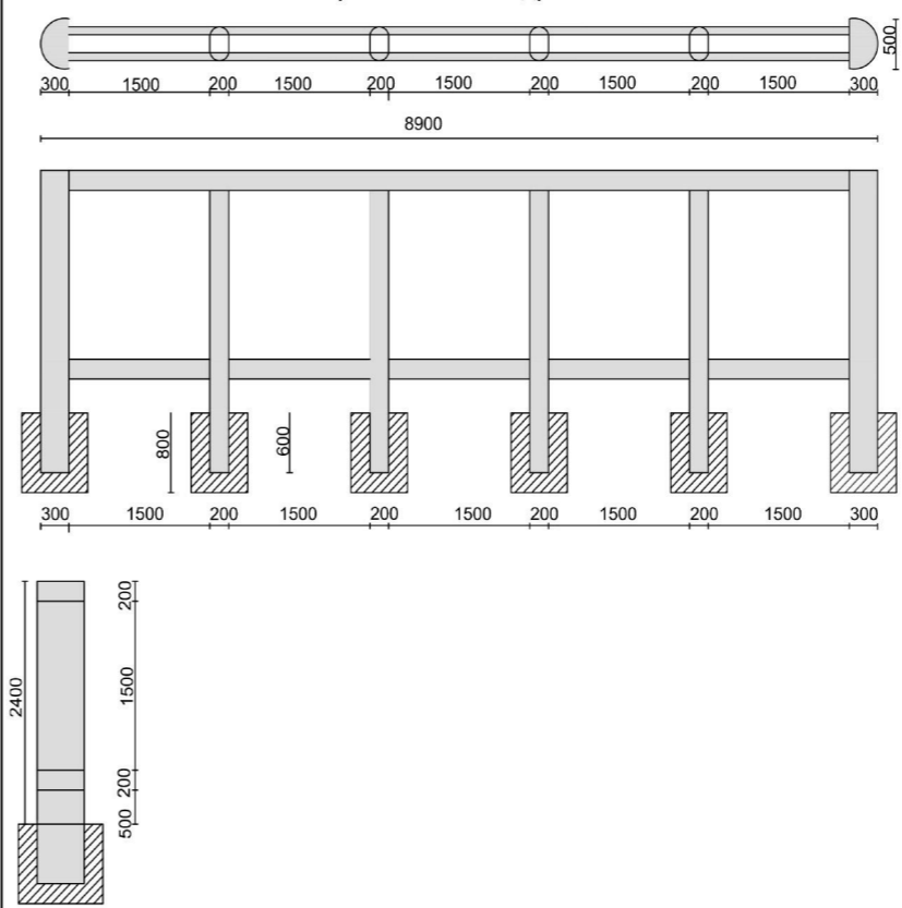
Технические характеристики рекламной конструкции (АФИШНЫЙ СТЕНД)
